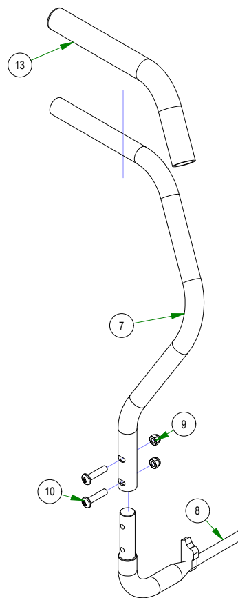
031-8850-70 ZT Steering Arm - Left
