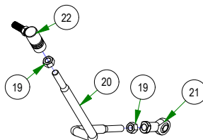
035-5450-00 Push Rod-Right
