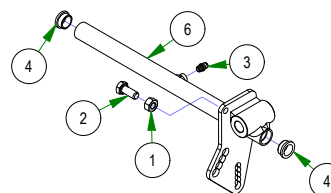
031-0054-21 2021 Maverick Drive Arm Actuator LH Assembly
